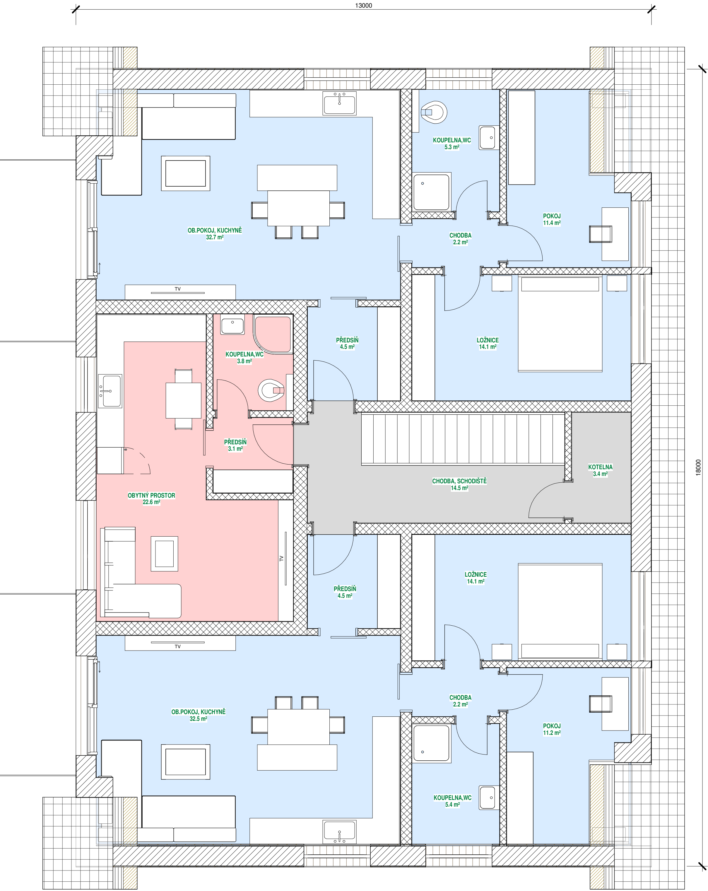
PŮDORYS 2NP
