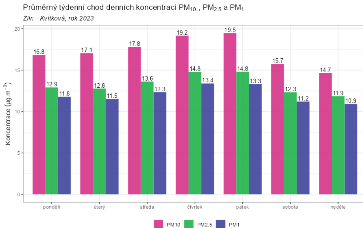
Obr. 20 – Průměrný týdenní chod denních koncentrací PM 10 , Zlín – Kvítková, rok 2023
