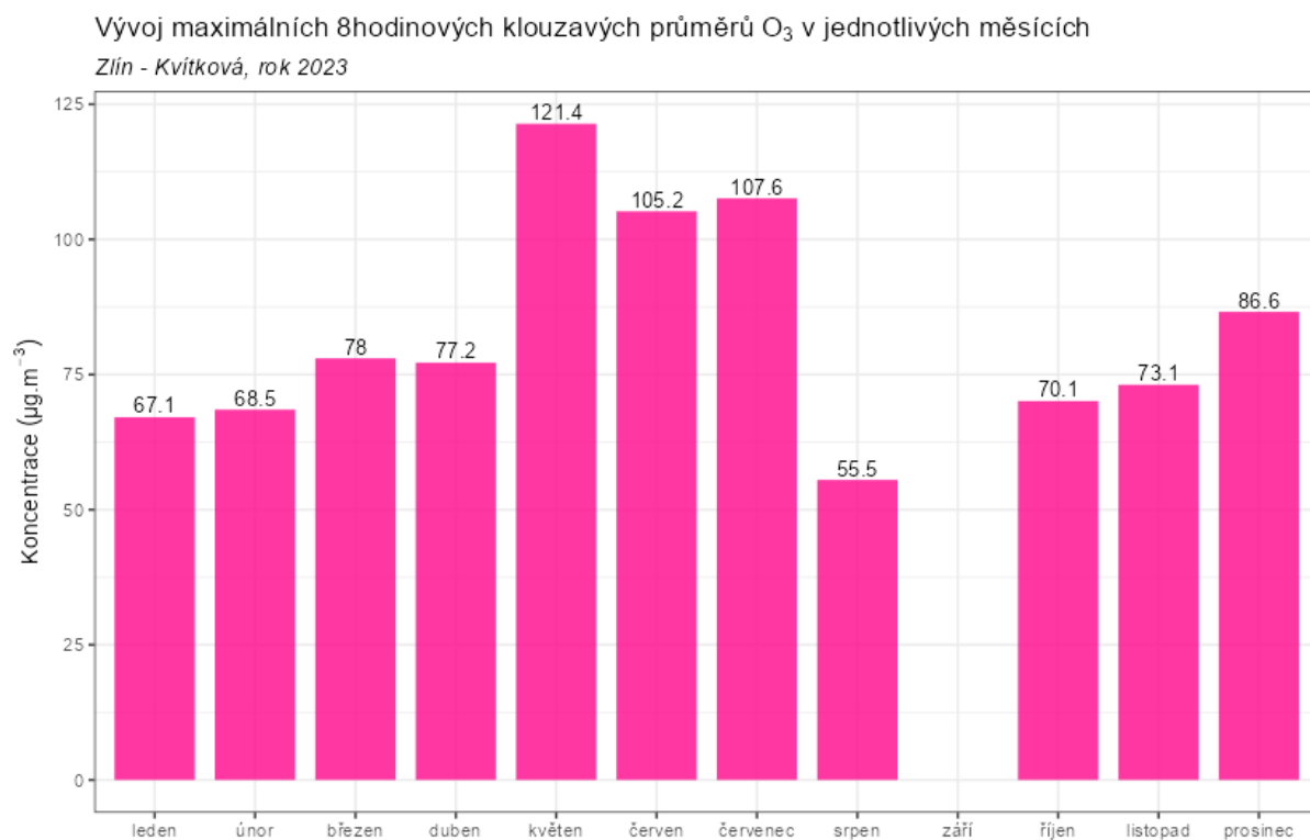
Obr. 55 – Maximální 8h klouzavé průměry O_3 za den v jednotlivých měsících, Zlín – Kvítková, rok 2023
