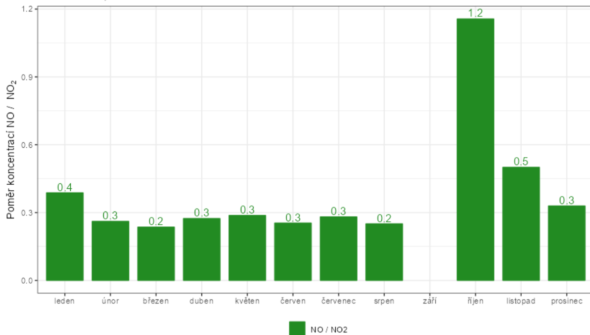
Obr. 39 – Poměr měsíčních koncentrací NO / NO 2 , lokalita Zlín – Kvítková, rok 2023
