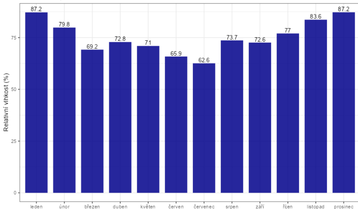
Obr. 7 – Průměrné měsíční relativní vlhkosti vzduchu, Zlín – Kvítková, rok 2023
