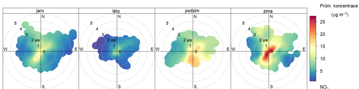
Obr. 47 – Koncentrační růžice jednotlivých ročních období, Zlín – Kvítková, rok 2023
