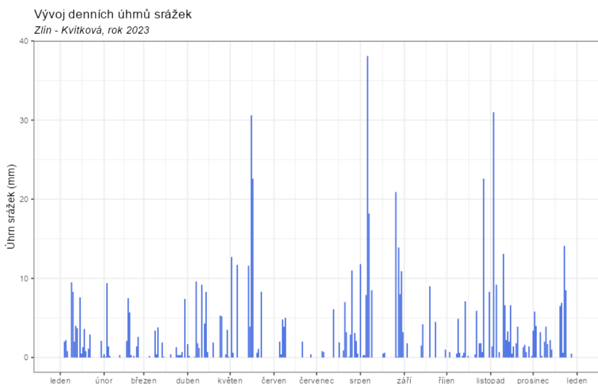
Obr. 8 – Denní úhrn srážek, Zlín – Kvítková, rok 2023
