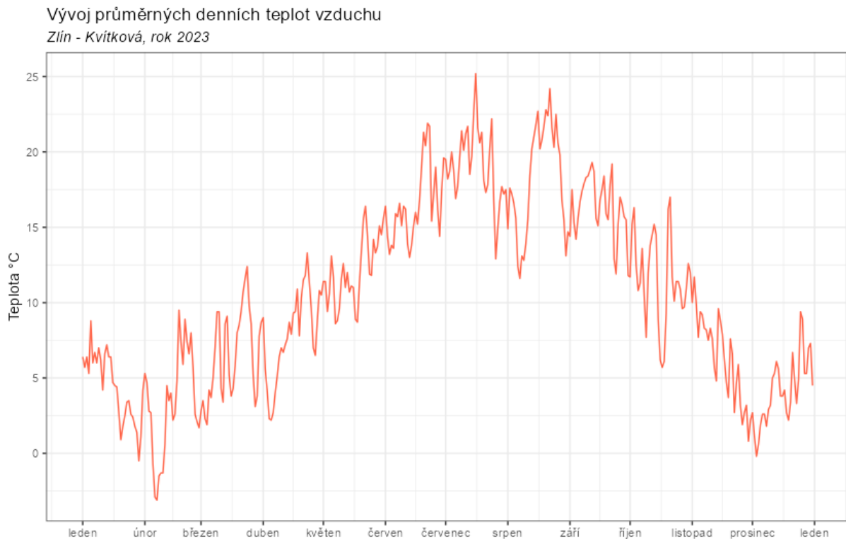
Obr. 4 – Průměrné denní teploty vzduchu, Zlín – Kvítková, rok 2023
