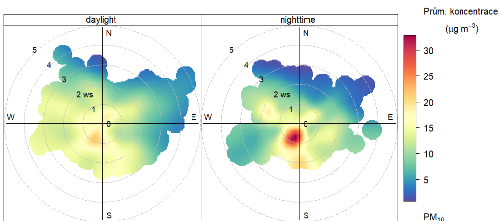
Obr. 23 – Koncentrační růžice ve dne (daytime) a v noci (nighttime), Zlín – Kvítková, rok 2023
