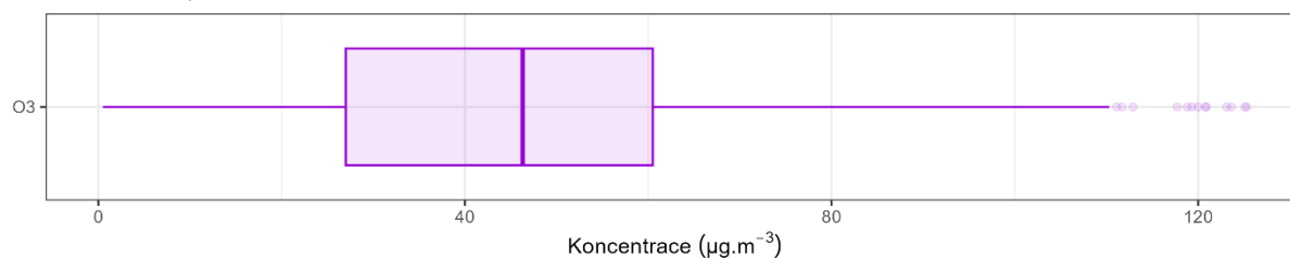
Obr. 54 – Statistické zpracování hodinových koncentrací O 3 v lokalitě Zlín – Kvítková, rok 2023
