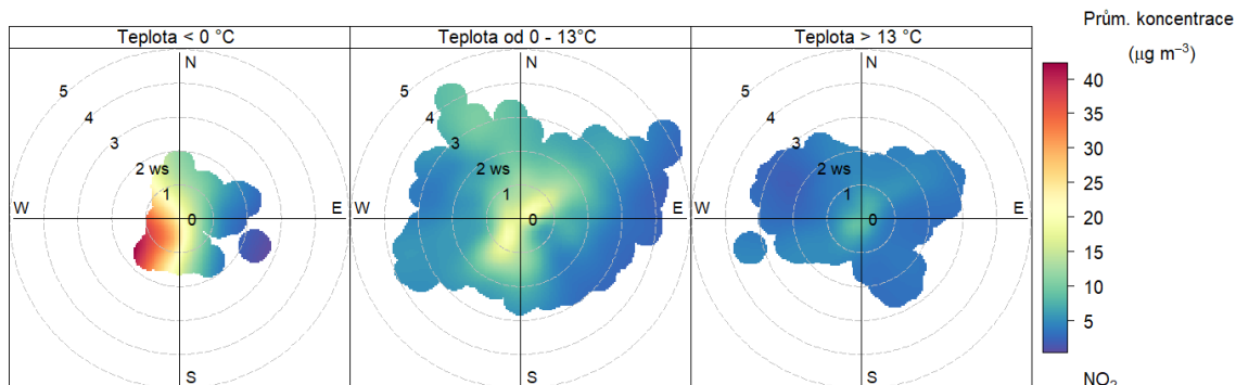
Obr. 48 – Koncentrační růžice členěná dle teplot, Zlín – Kvítková, rok 2023
