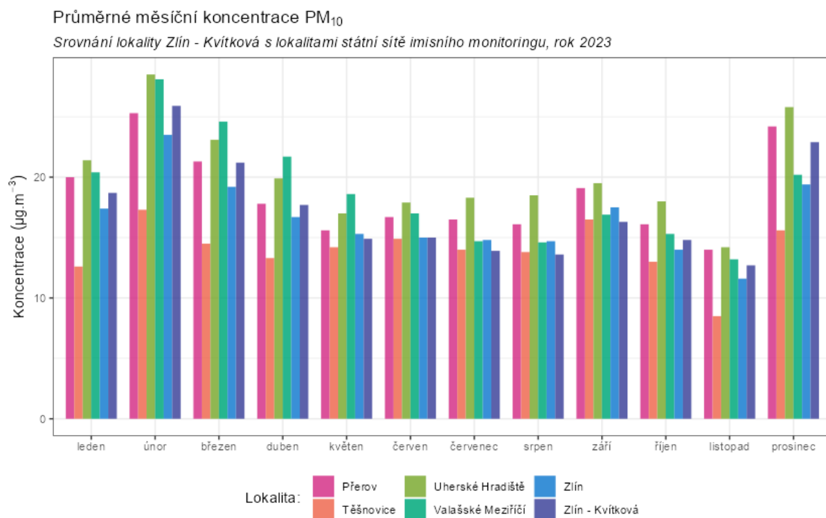
Obr. 31 – Srovnání průměrných měsíčních koncentrací PM_{10} lokality Zlín – Kvítková s okolními stanicemi státní sítě imisního monitoringu, rok 2023
