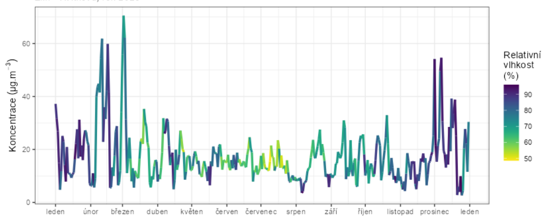
Obr. 19 – Vliv teploty (nahore), rychlosti větru (uprostřed) a relativní vlhkosti (dole) na koncentrace PM 10 , Zlín – Kvítková, rok 2023
