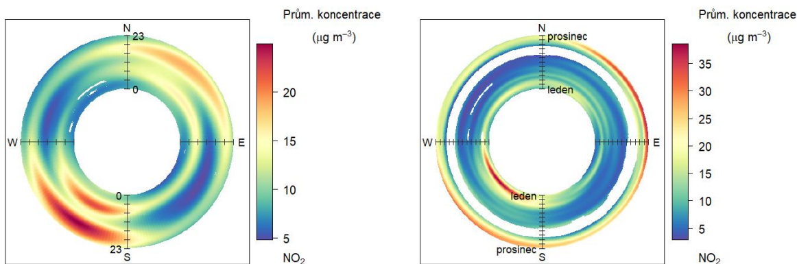
Obr. 49 – Průměrný denní chod (vlevo) a roční chod (vpravo) koncentrací dle směru větru, Zlín – Kvítková, rok 2023
