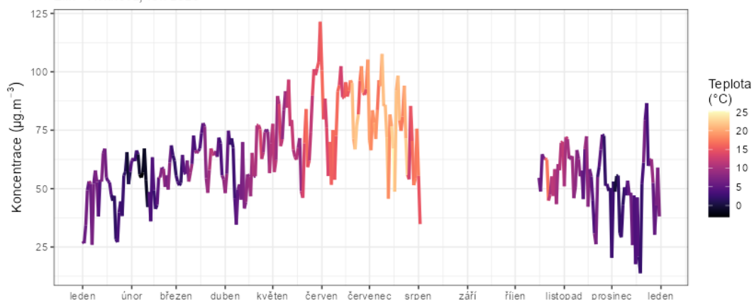
Vývoj maximálních 8h koncentrací O 3 za den v závislosti na teplotě vzduchu
