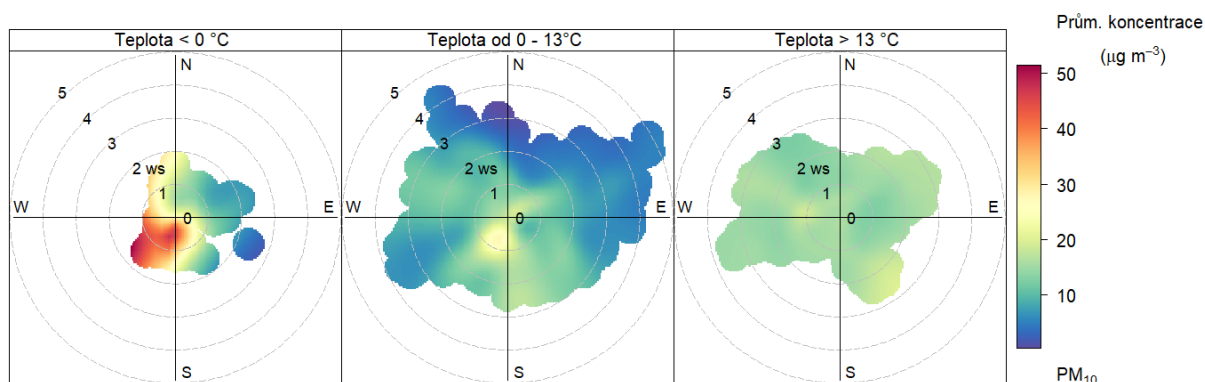
Obr. 26 – Koncentrační růžice členěná dle teplot, Zlín – Kvítková, rok 2023
