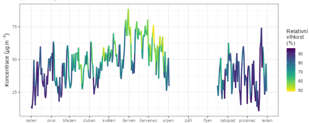
Obr. 57 – Vliv teploty (nahore), rychlosti větru (uprostřed) a relativní vlhkosti (dole) na koncentrace O 3 , Zlín – Kvítková, rok 2023
