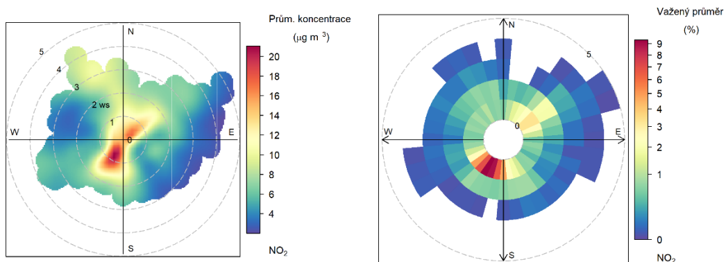
Obr. 44 – Koncentrační růžice (vlevo) a vážená koncentrační růžice (vpravo) pro NO 2 , Zlín – Kvítková, rok 2023
