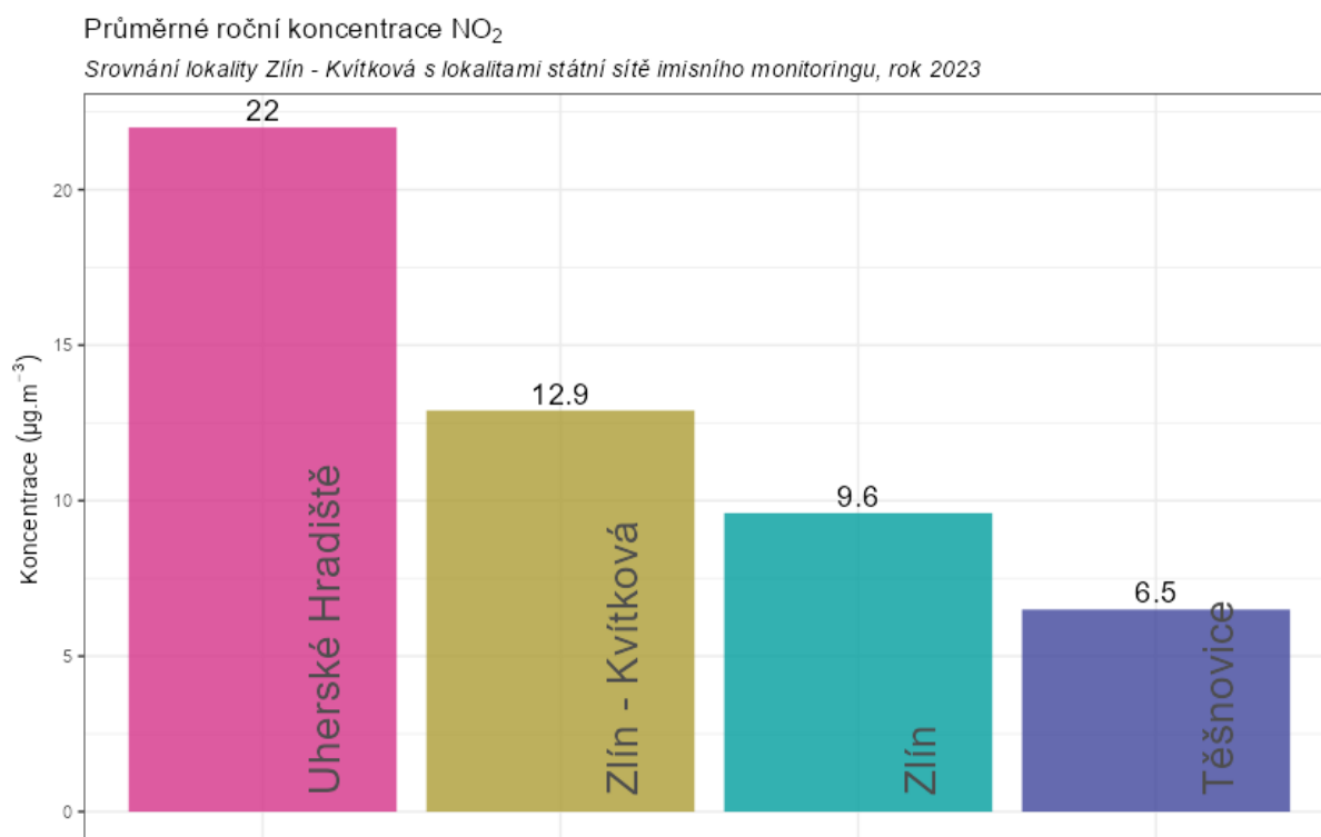
Obr. 50 – Srovnání průměrné roční koncentrace NO 2 lokality Zlín – Kvítková s okolními stanicemi státní sítě imisního monitoringu, rok 2023
