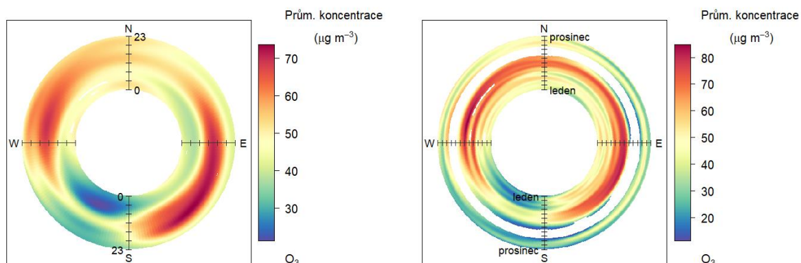
Obr. 64 – Průměrný denní chod (vlevo) a roční chod (vpravo) koncentrací dle směru větru, Zlín – Kvítková, rok 2023
