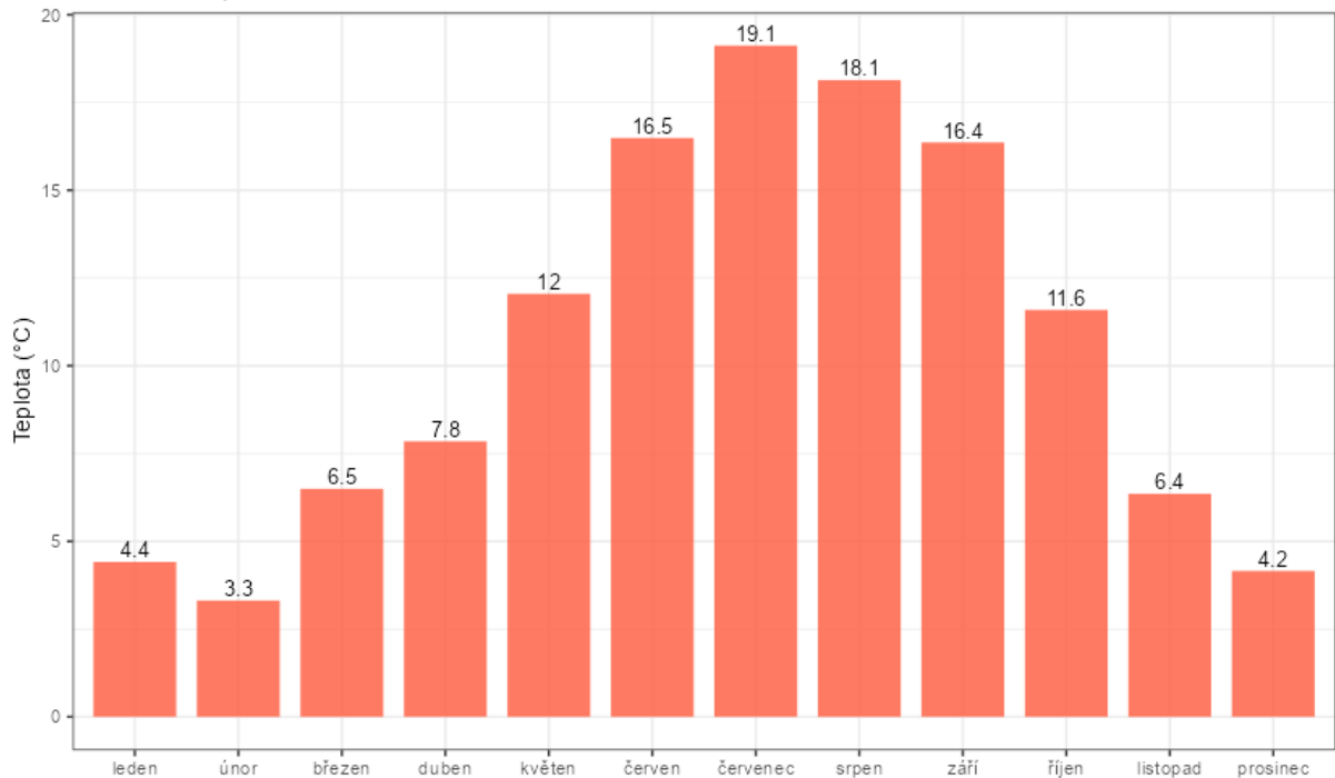
Vývoj průměrných měsíčních teplot vzduchu Zlín - Kvítková, rok 2023
