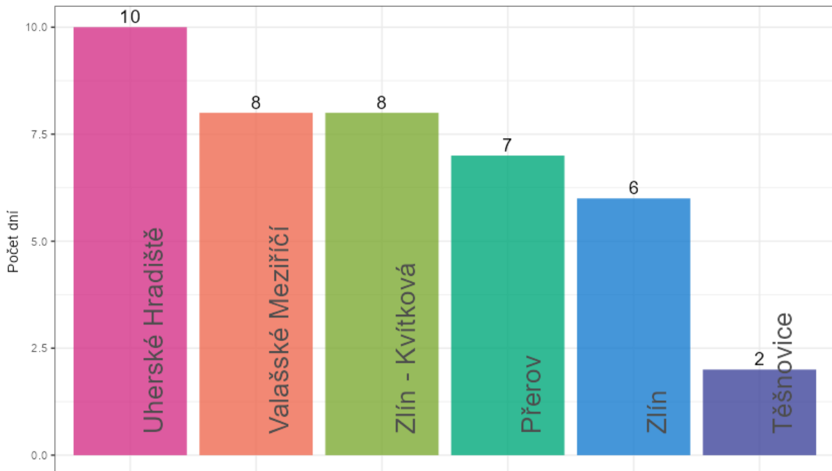
Obr. 30 – Počet dní s průměrnými denními koncentracemi PM 10 vyššími, než je hodnota imisního limitu pro průměrnou denní koncentraci PM 10 , vybrané lokality Olomouckého kraje, rok 2023
