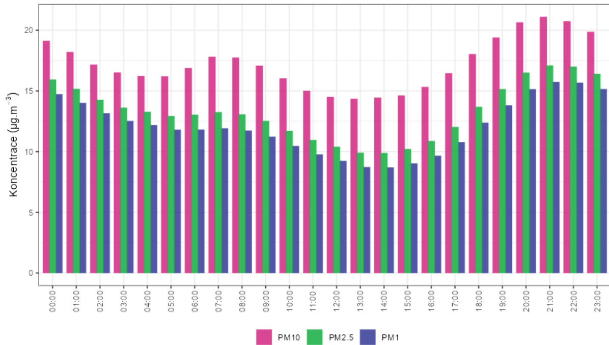
Průměrný denní chod hodinových koncentrací PM 10 , PM 2.5 a PM 1 Zlín - Kvítková, rok 2023
