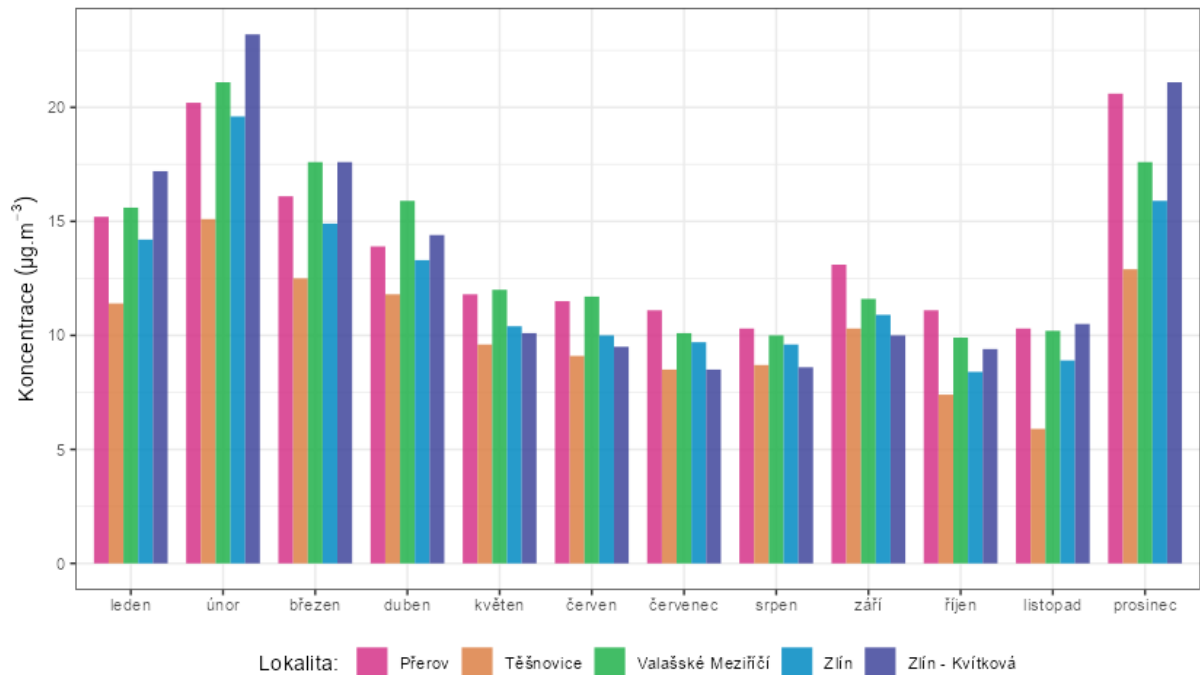
Obr. 32 – Srovnání průměrných měsíčních koncentrací PM 2.5 lokality Zlín – Kvítková s okolními stanicemi státní sítě imisního monitoringu, rok 2023
