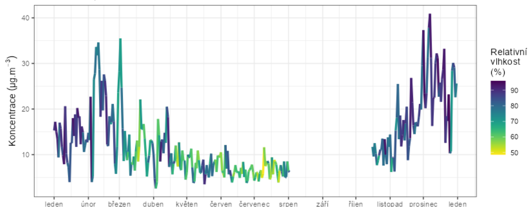
Obr. 41 – Vliv teploty (nahore), rychlosti větru (uprostřed) a relativní vlhkosti (dole) na koncentrace NO 2 , Zlín – Kvítková, rok 2023
