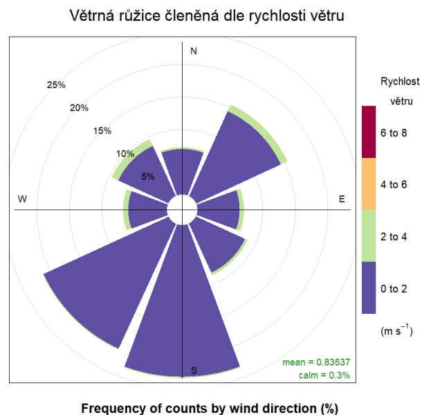
Obr. 1 – Větrná růžice členěná dle rychlosti větru, Zlín – Kvítková, rok 2023
