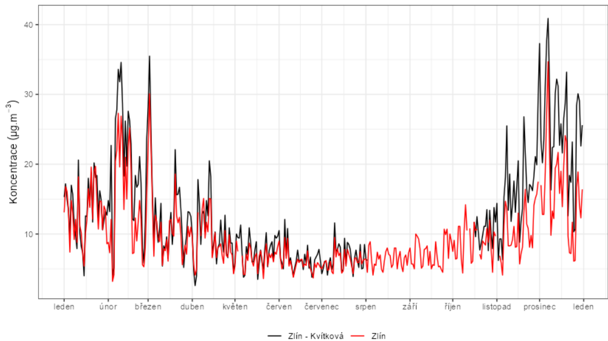
Obr. 52 – Srovnání průměrných denních koncentrací NO 2 , lokality Zlín – Kvítková a Zlín, rok 2023
