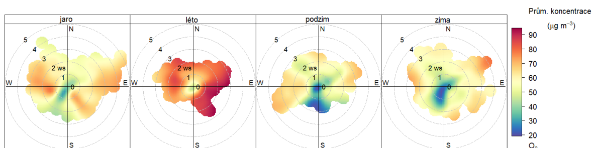
Obr. 62 – Koncentrační růžice jednotlivých ročních období, Zlín – Kvítková, rok 2023
