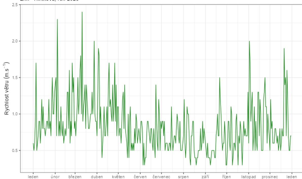
Obr. 2 – Průměrné denní rychlosti větru, Zlín – Kvítková, rok 2023
