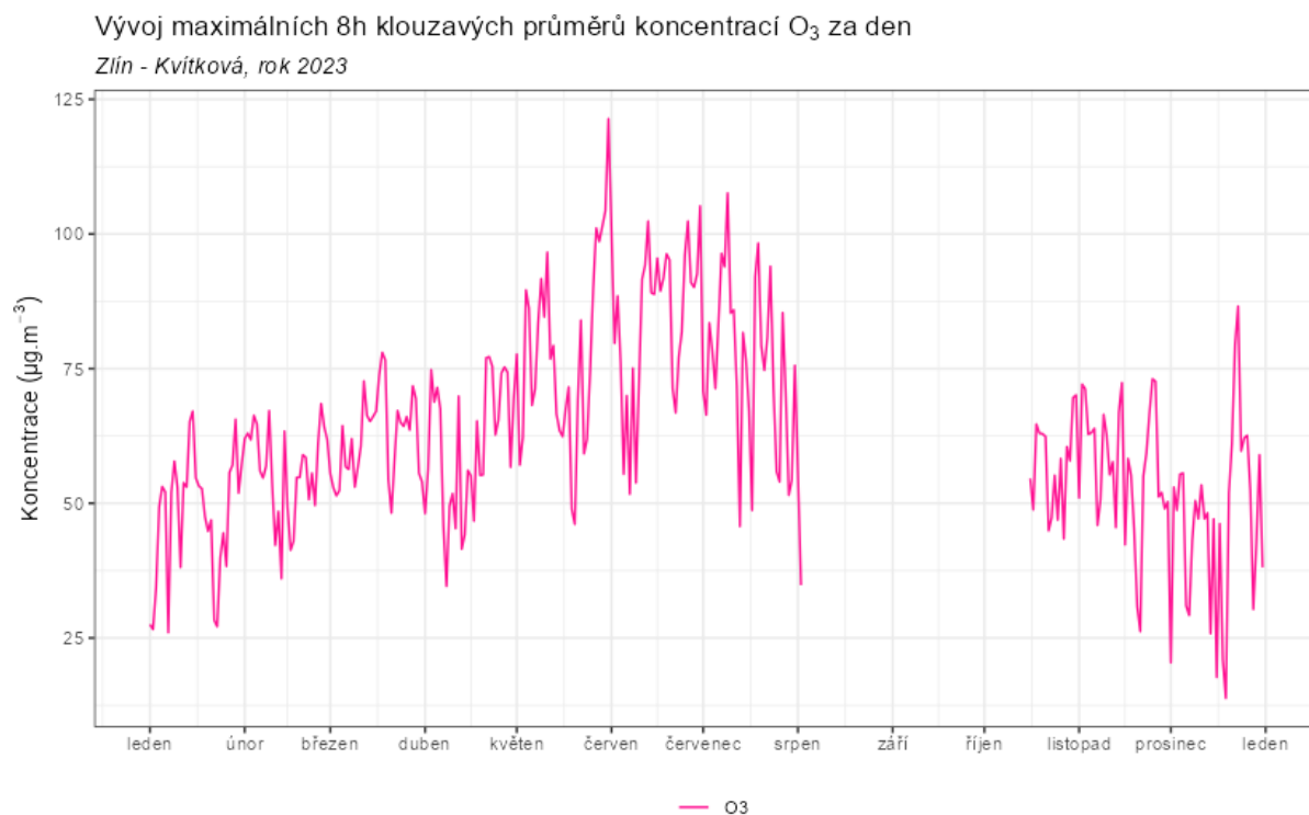
Obr. 56 – Vývoj maximálních 8h klouzavých průměrů O 3 za den, Zlín – Kvítková, rok 2023
