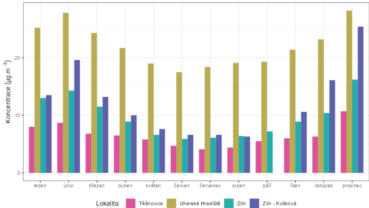
Obr. 51 – Srovnání průměrných měsíčních koncentrací NO 2 lokality Zlín – Kvítková s okolními stanicemi státní sítě imisního monitoringu, rok 2023
