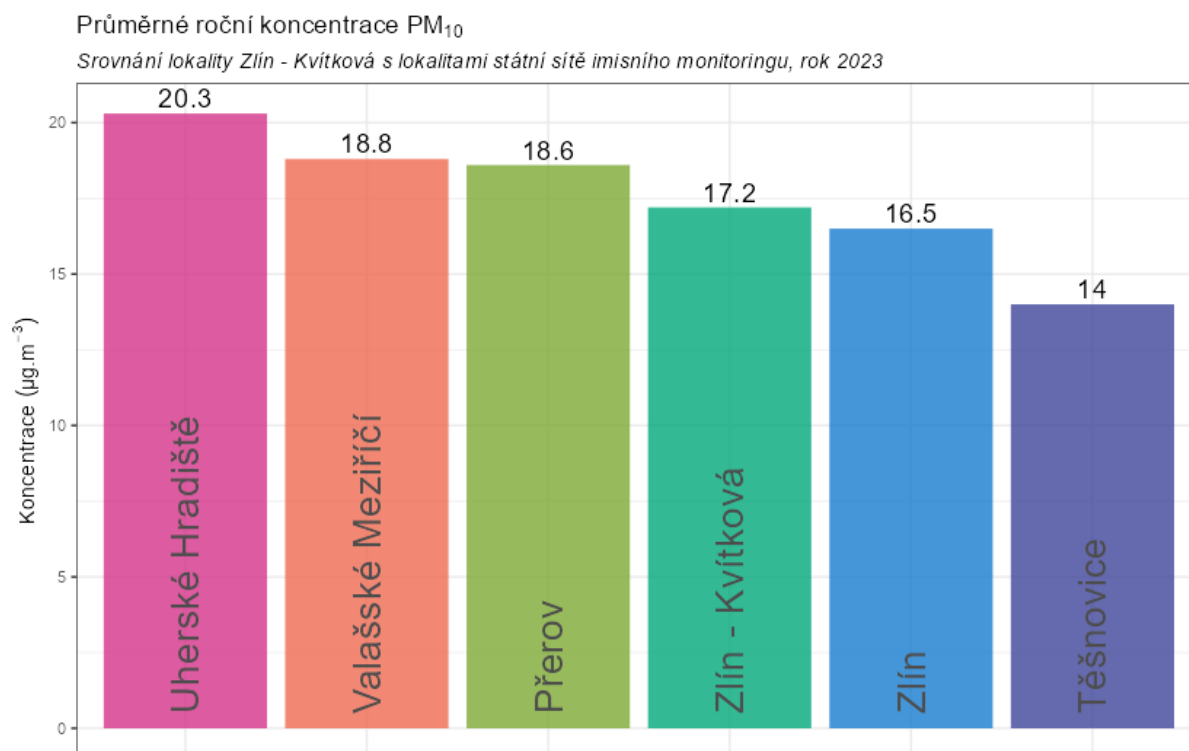
Obr. 28 – Srovnání průměrné roční koncentrace PM 10 lokality Zlín – Kvítková s okolními stanicemi státní sítě imisního monitoringu, rok 2023
