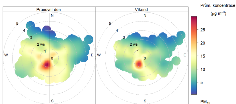
Obr. 24 – Koncentrační růžice v pracovní dny a o víkendu, Otrokovice – město, rok 2023
