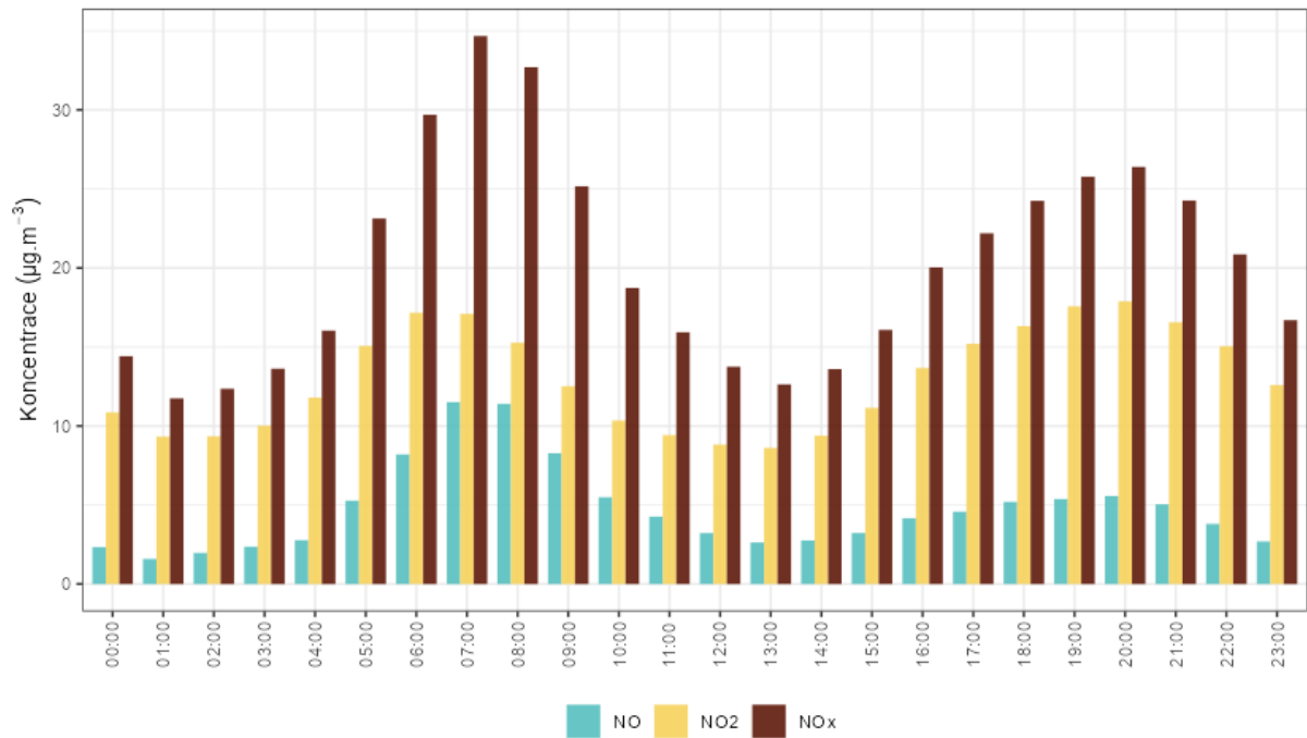
Obr. 43 – Denní chod hodinových koncentrací NO 2 , Zlín – Kvítková, rok 2023
