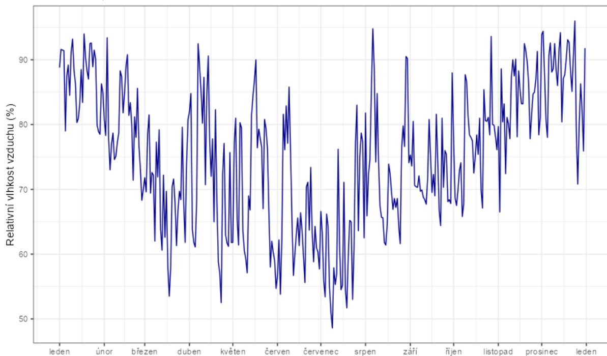
Obr. 6 - Průměrné denní relativní vlhkosti vzduchu, Zlín – Kvítková, rok 2023
