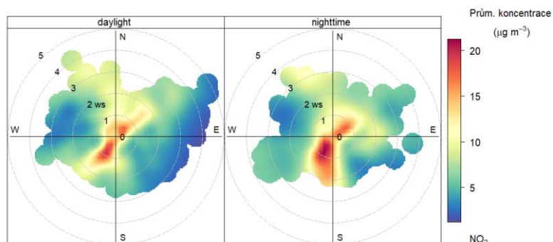
Obr. 45 - Koncentrační růžice ve dne (daytime) a v noci (nighttime), Zlín – Kvítková, rok 2023
