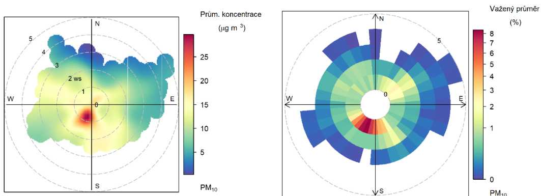
Obr. 22 – Koncentrační růžice (vlevo) a vážená koncentrační růžice (vpravo) pro PM_{10} , Zlín – Kvítková, rok 2023
