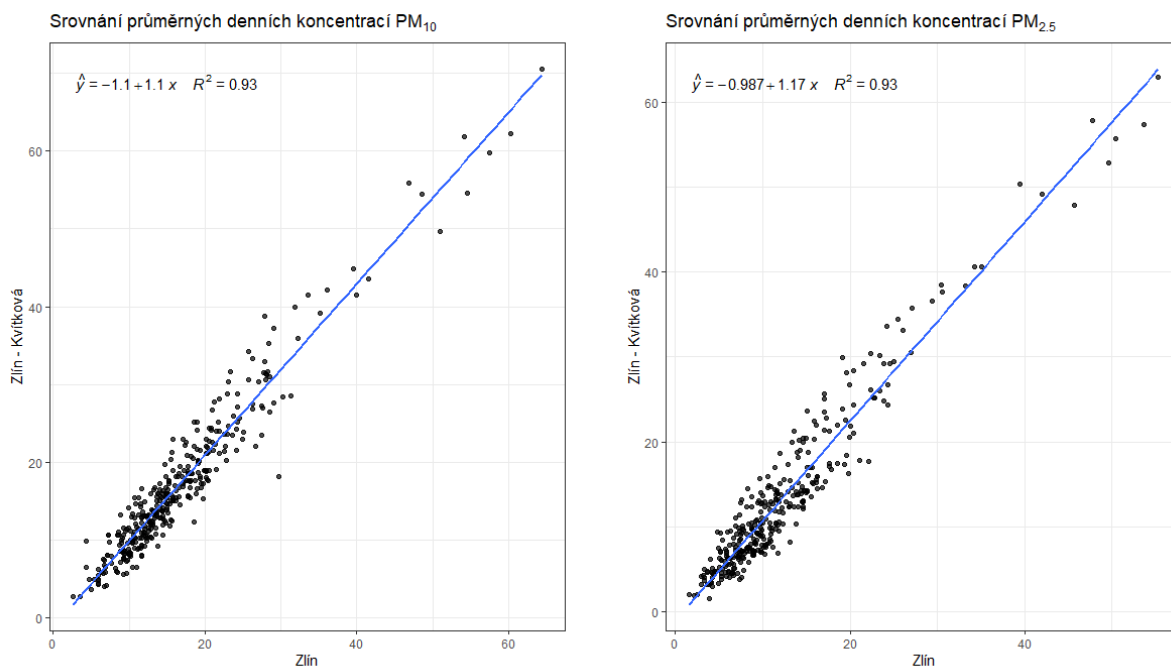
Obr. 34 – Srovnání průměrných denních koncentrací v lokalitě Zlín a Zlín – Kvítková, rok 2023
