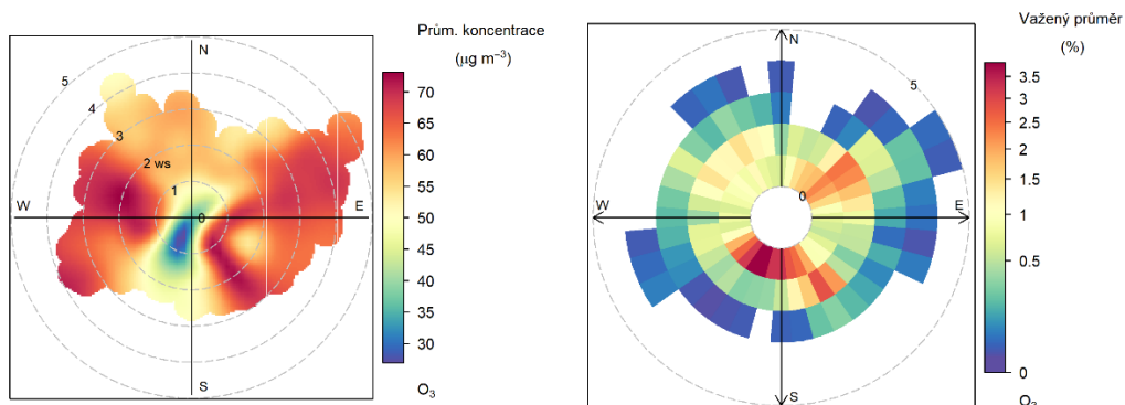
Obr. 60 – Koncentrační růžice (vlevo) a vážená koncentrační růžice (vpravo) pro O 3 , Zlín – Kvítková, rok 2023
