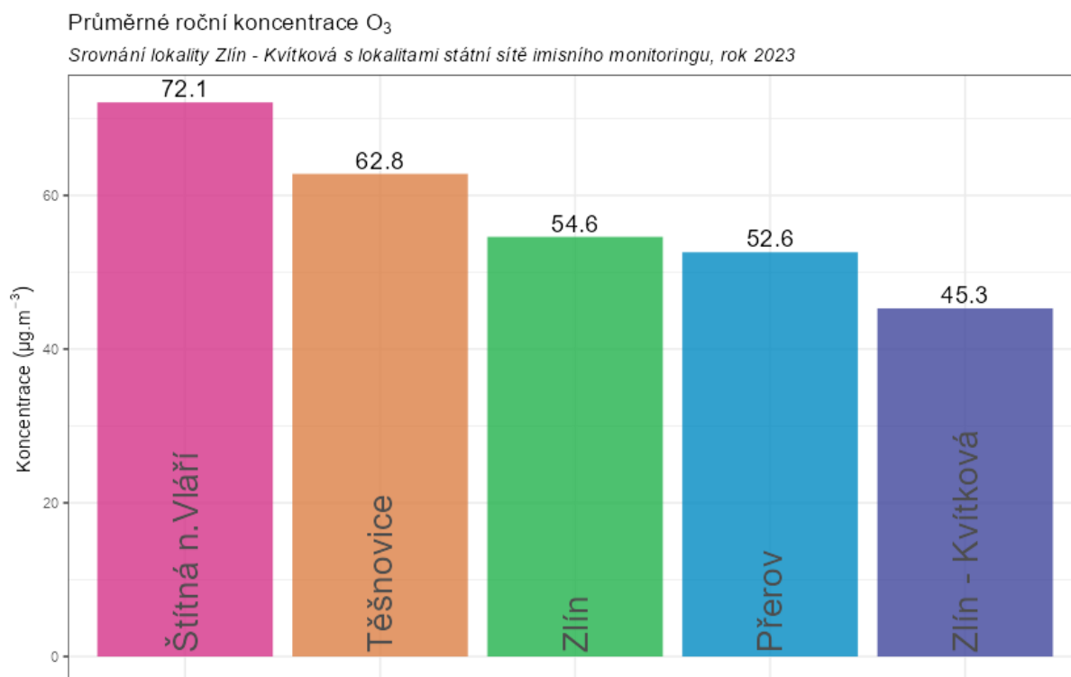
Obr. 65 – Srovnání průměrné roční koncentrace O_3 lokality Zlín – Kvítková s okolními stanicemi státní sítě imisního monitoringu, rok 2023
