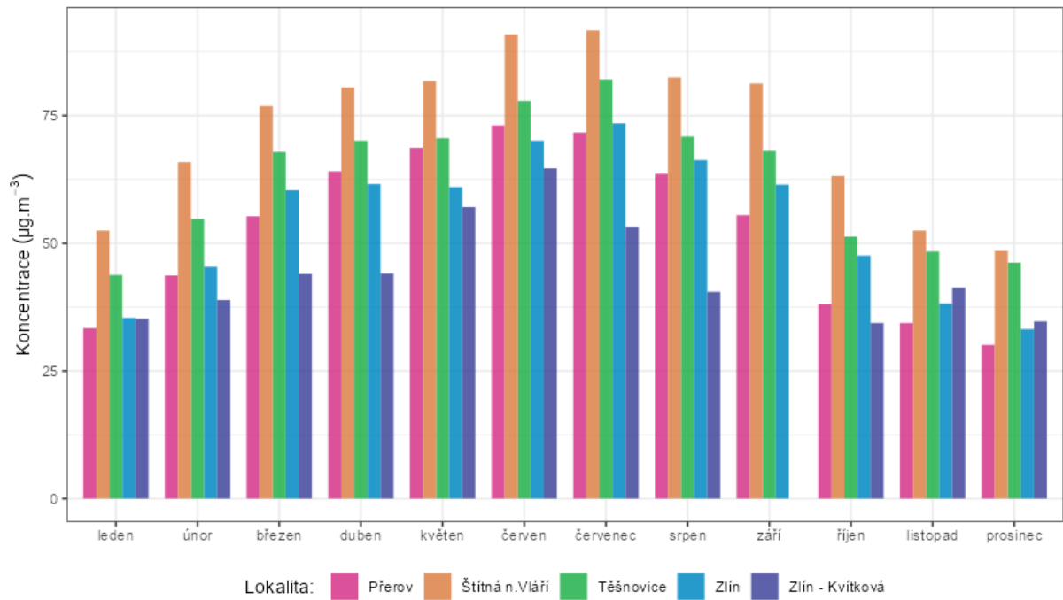
Obr. 66 – Srovnání průměrných měsíčních koncentrací O 3 lokality Zlín – Kvítková s okolními stanicemi státní sítě imisního monitoringu, rok 2023
