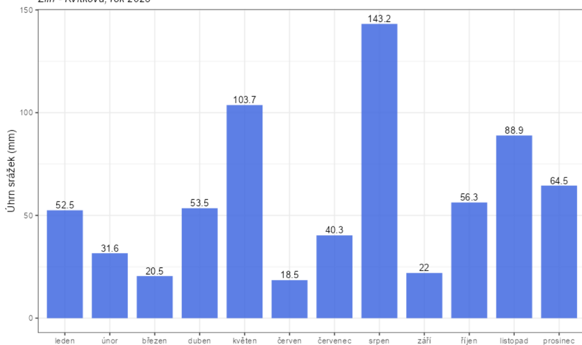
Obr. 9 – Měsíční úhrn srážek, Zlín – Kvítková, rok 2023
