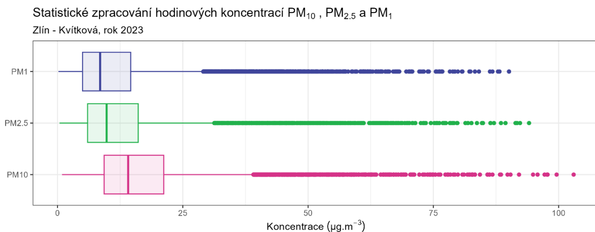
Obr. 13 – Statistické zpracování hodinových koncentrací PM 10 , PM 2,5 a PM 1 v lokalitě Zlín – Kvítková, rok 2023
