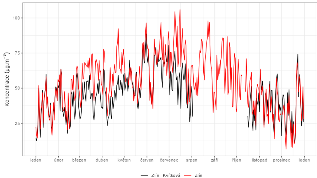
Obr. 67 – Srovnání průměrných denních koncentrací O 3 , lokality Zlín – Kvítková a Zlín, rok 2023
