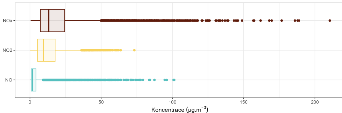
Statistické zpracování hodinových koncentrací NO, NO 2 a NO x Zlín - Kvítková, rok 2023
