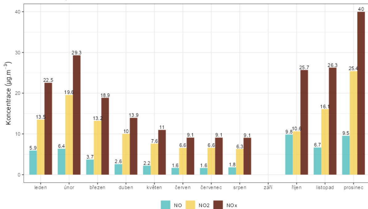
Obr. 38 - Průměrné měsíční koncentrace NO, NO 2 a NO x , Zlín – Kvítková, rok 2023
