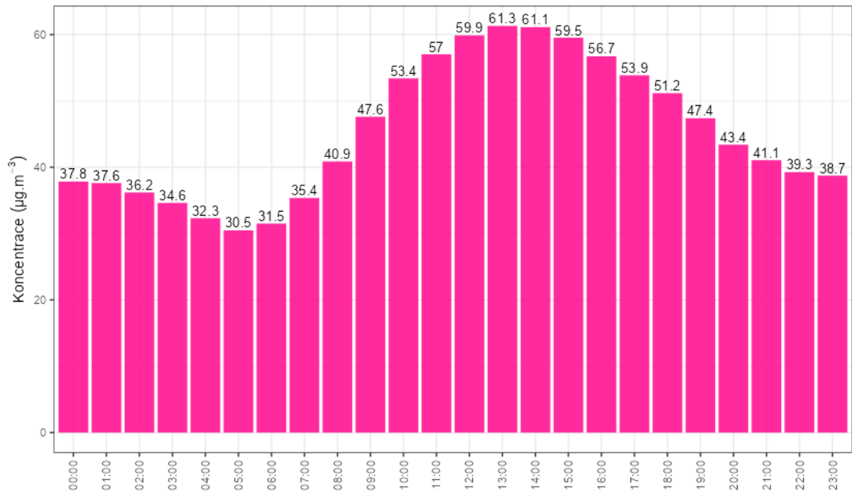
Obr. 59 – Denní chod hodinových koncentrací O 3 , Zlín – Kvítková, rok 2023
