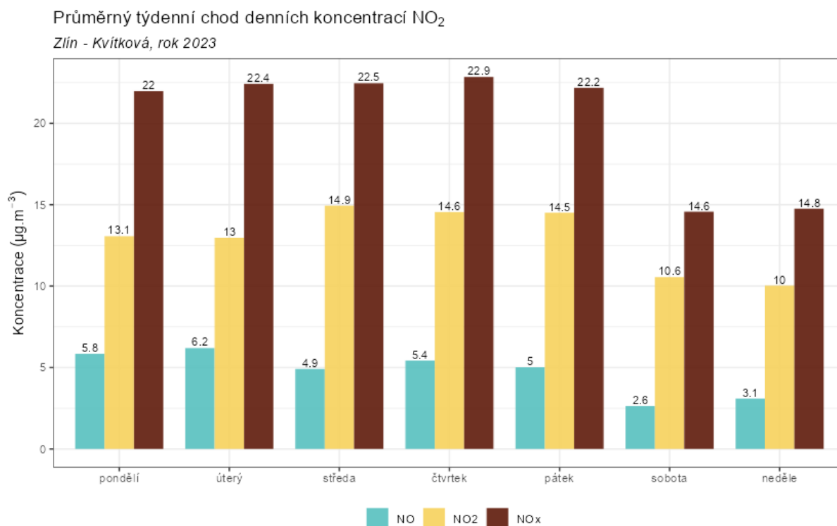
Obr. 42 – Průměrný týdenní chod denních koncentrací NO 2 , Zlín – Kvítková, rok 2023
