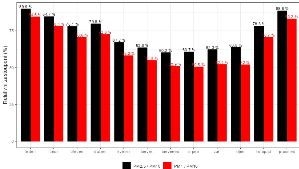
Obr. 15 – Průměrné měsíční zastoupení PM 2,5 v PM 10 a PM 1 v PM 10 , lokalita Zlín – Kvítková, rok 2023
