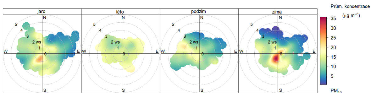
Obr. 25 – Koncentrační růžice jednotlivých ročních období, Zlín – Kvítková, rok 2023
