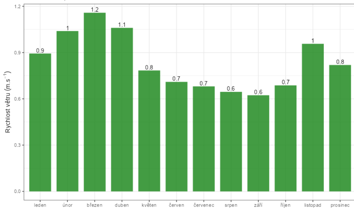
Obr. 3 – Průměrné měsíční rychlosti větru, Zlín – Kvítková, rok 2023
