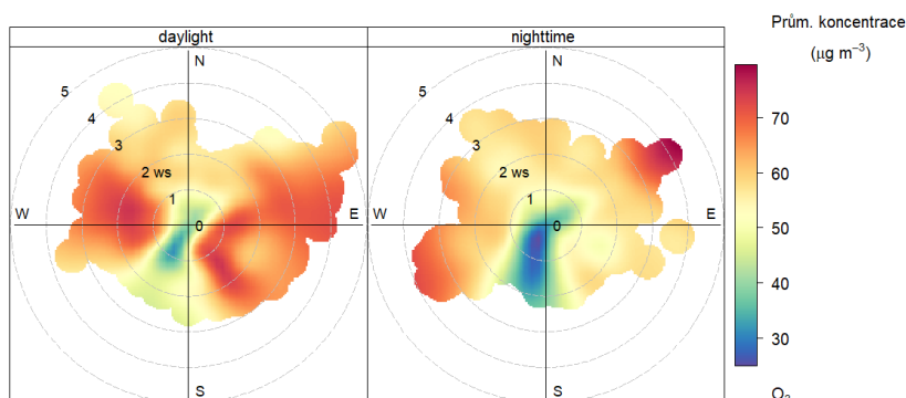
Obr. 61 - Koncentrační růžice ve dne (daytime) a v noci (nighttime), Zlín – Kvítková, rok 2023
