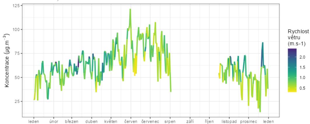
Vývoj maximálních 8h koncentrací O 3 za den v závislosti na rychlosti větru
