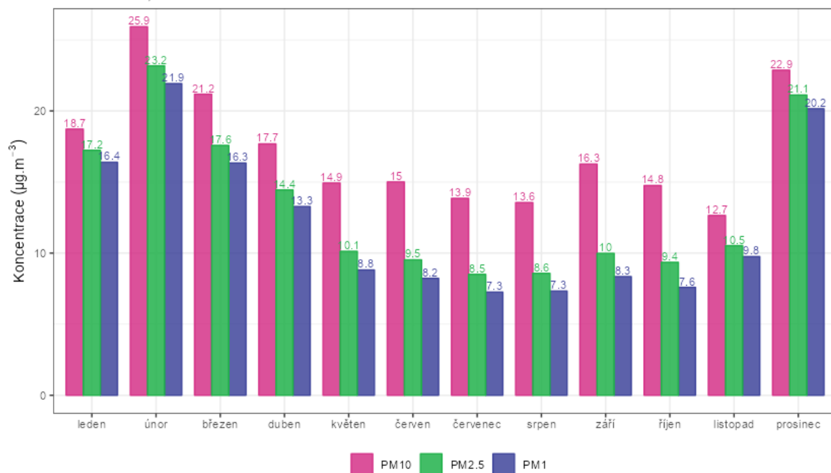
Obr. 14 - Průměrné měsíční koncentrace PM 10 , PM 2,5 a PM 1 , Zlín – Kvítková, rok 2023
