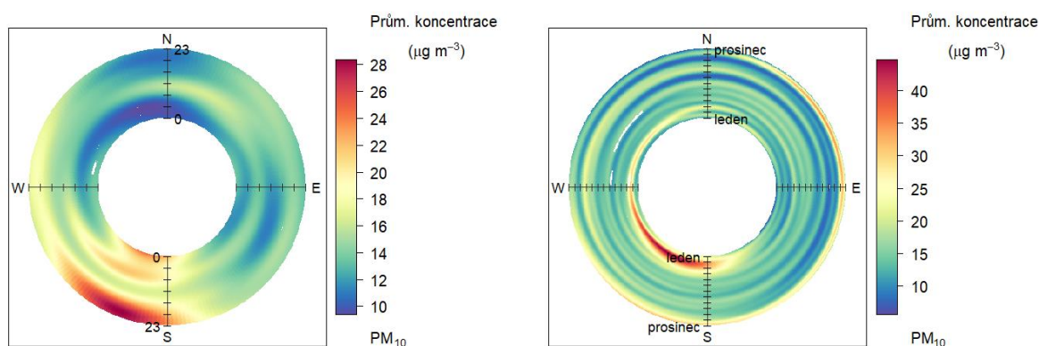
Obr. 27 – Průměrný denní chod (vlevo) a roční chod (vpravo) koncentrací dle směru větru, Zlín – Kvítková, rok 2023
