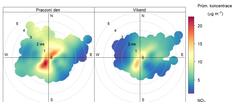
Obr. 46 – Koncentrační růžice NO 2 v pracovní dny a o víkendu, lokalita Zlín – Kvítková, rok 2023
