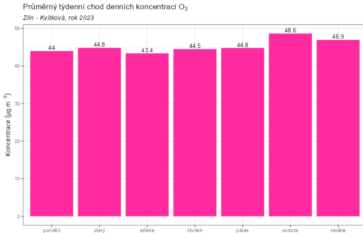
Obr. 58 - Průměrný týdenní chod denních koncentrací O 3 , Zlín – Kvítková, rok 2023
