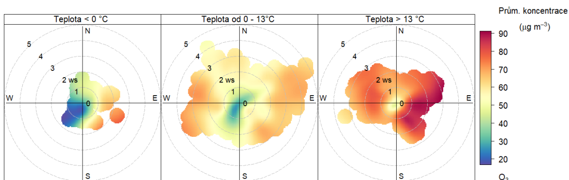
Obr. 63 – Koncentrační růžice členěná dle teplot, Zlín – Kvítková, rok 2023
