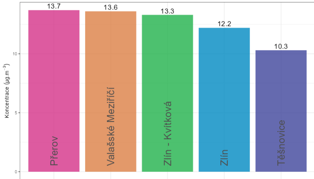
Obr. 29 – Srovnání průměrné roční koncentrace PM 2,5 lokality Zlín – Kvítková s okolními stanicemi státní sítě imisního monitoringu, rok 2023
